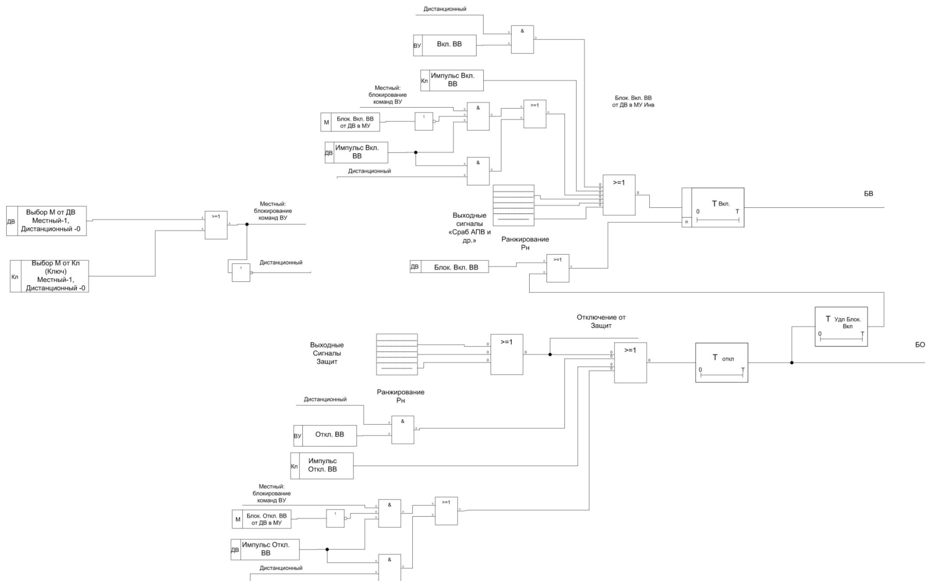
Рис.1.7.13 Функциональная схема блоков включения и отключения
