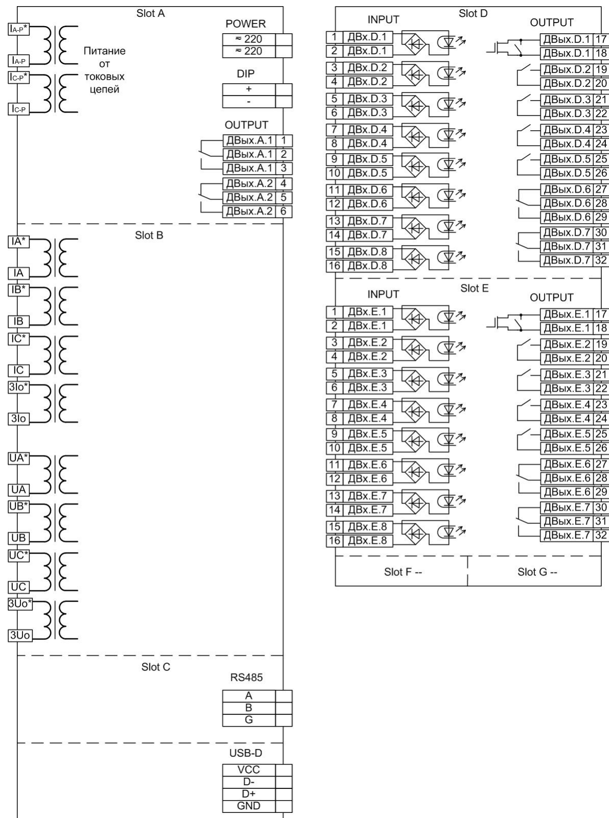
Рис. 2.1.4 Упрощенная схема подключения MZD-F (аппаратная конфигурация G)
