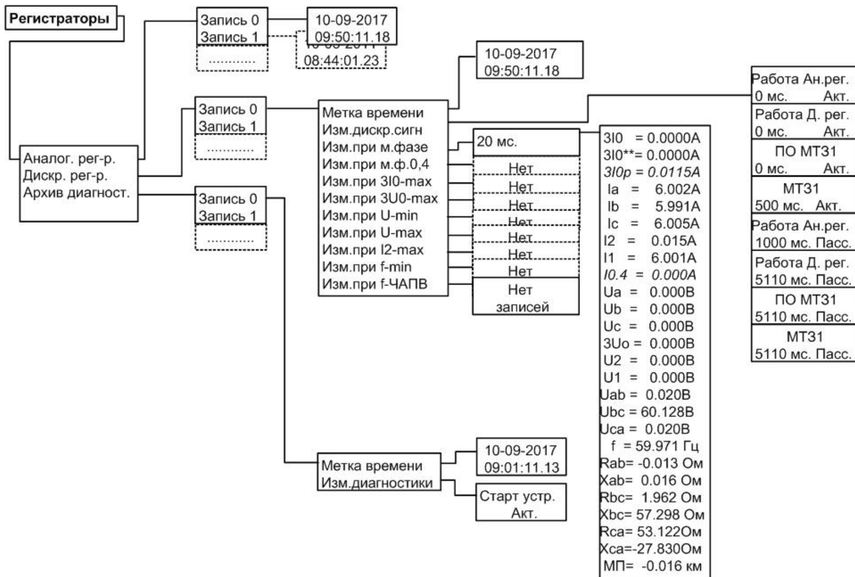
Рис. 3.8 Структура пункта меню "Регистраторы"
