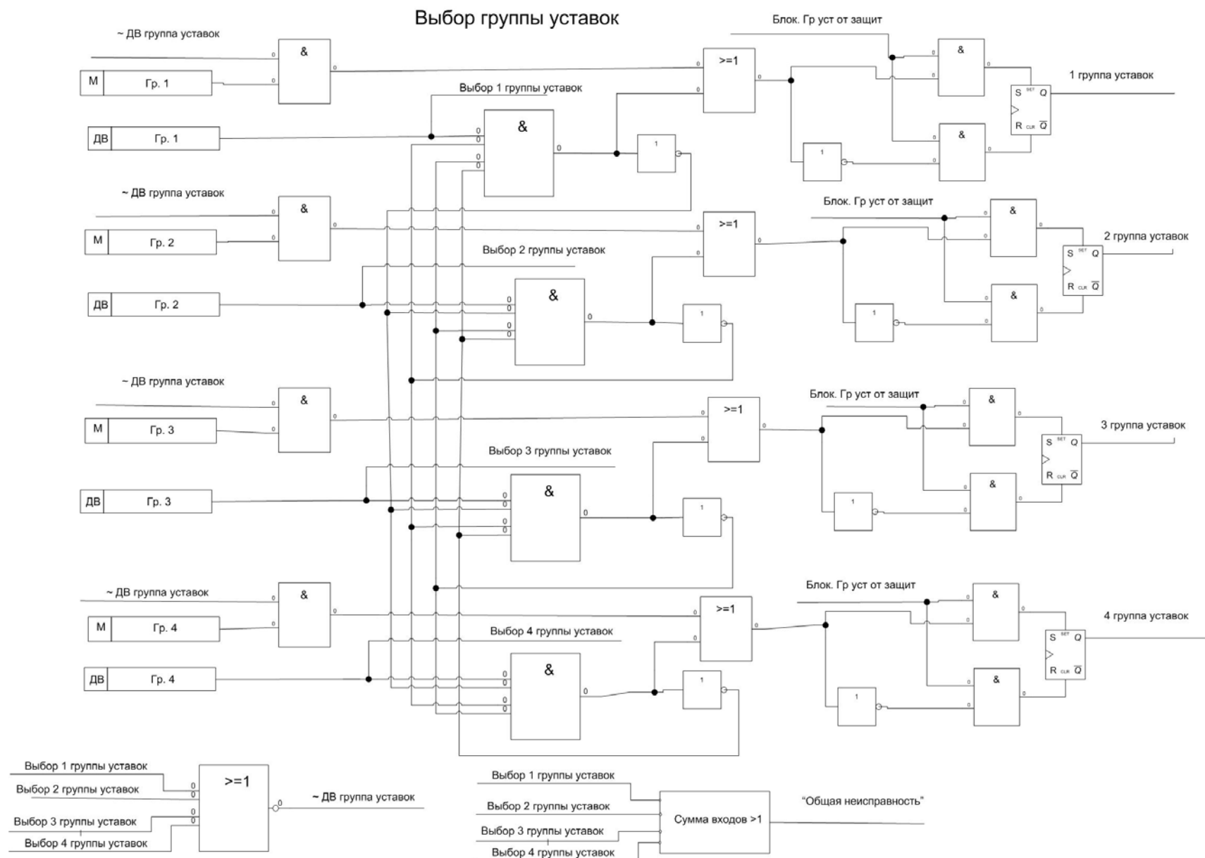
Рис. 1.7.1.1 Функциональная схема выбора группы уставок (начало)
