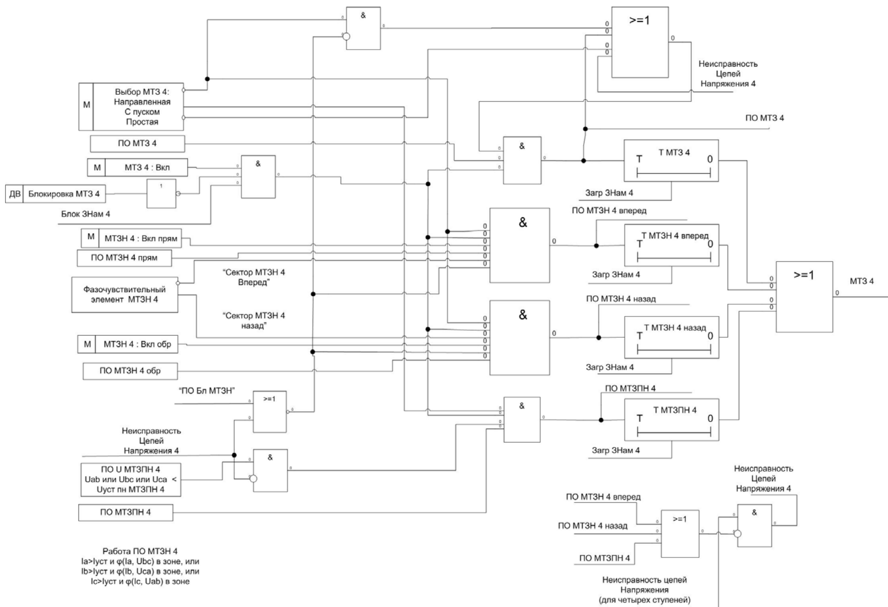
Рис. 1.7.2.6 Функциональная схема блока МТЗ4
