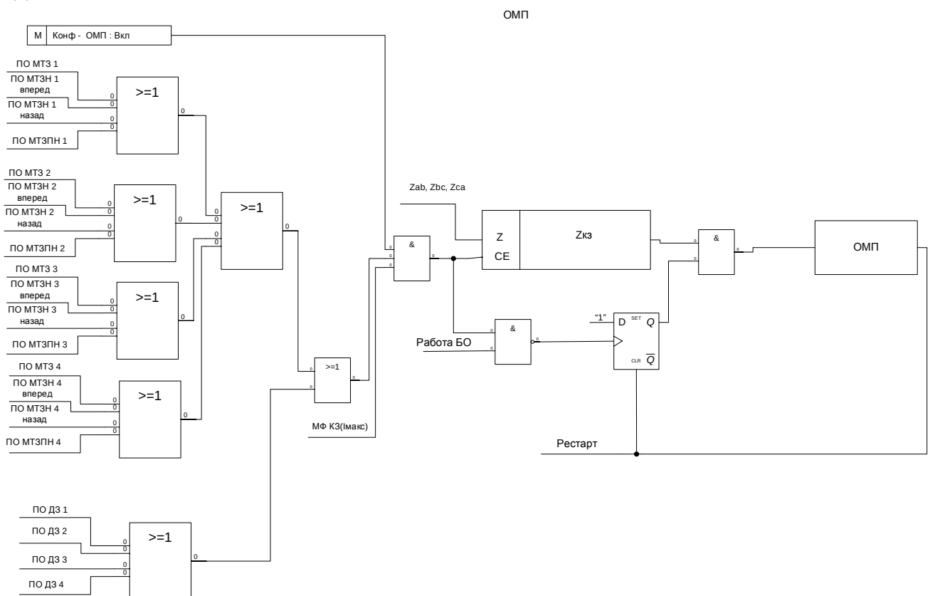
Рис. 1.7.23 Функциональная схема блока определения места повреждения
