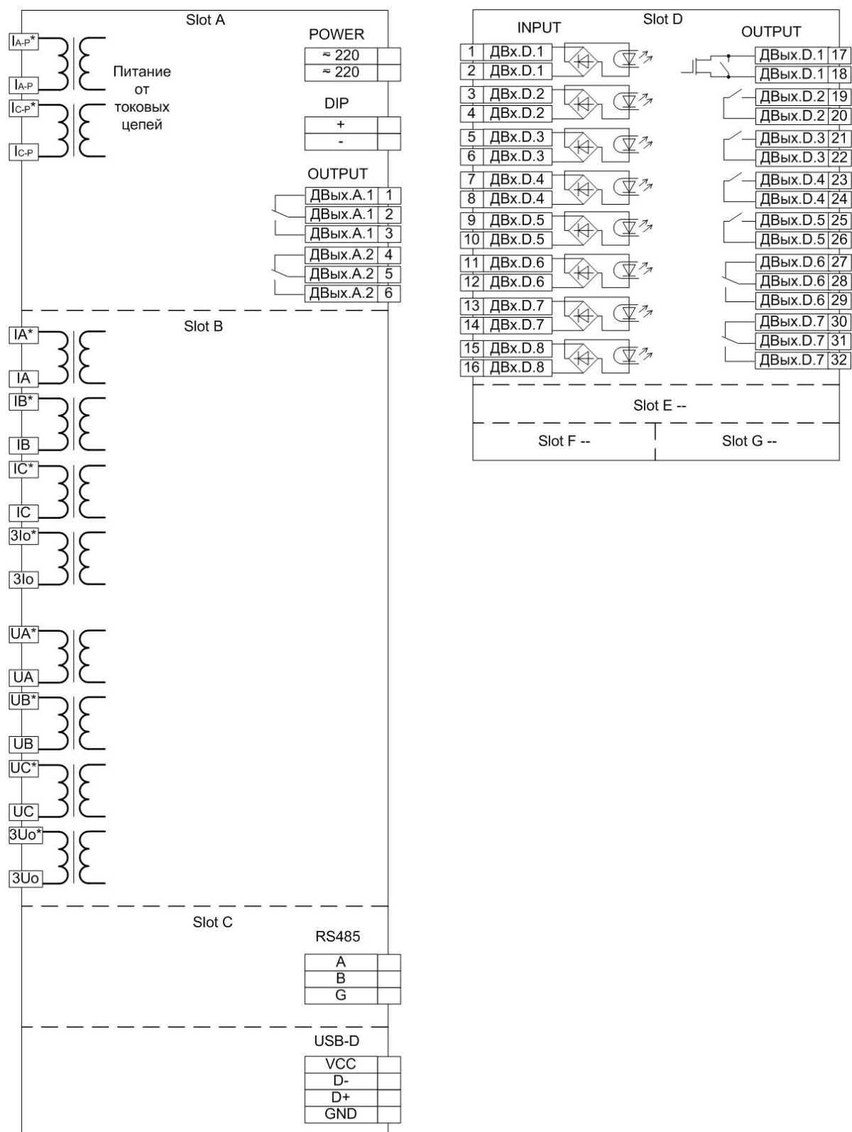
Рис. 2.1.1 Упрощенная схема подключения MZD-F (аппаратная конфигурация А)
