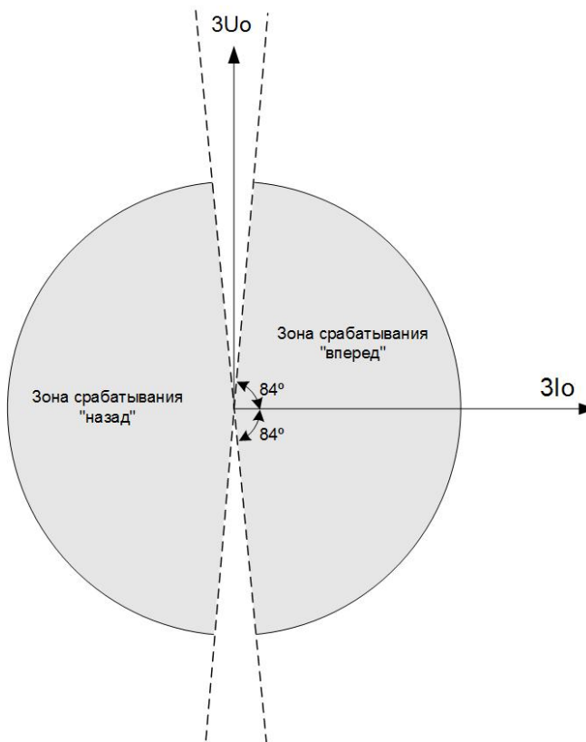
Рис. 1.7.4.1 Диаграмма направленности НЗЗ
