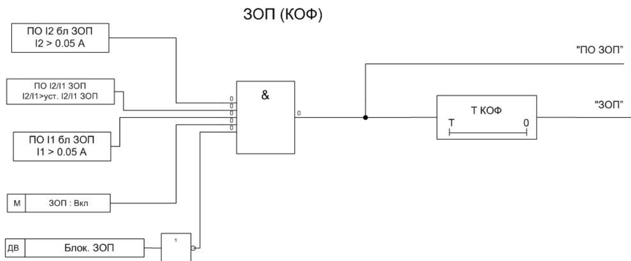
Рис. 1.7.8 Функциональная схема блока ЗОП(КОФ)
