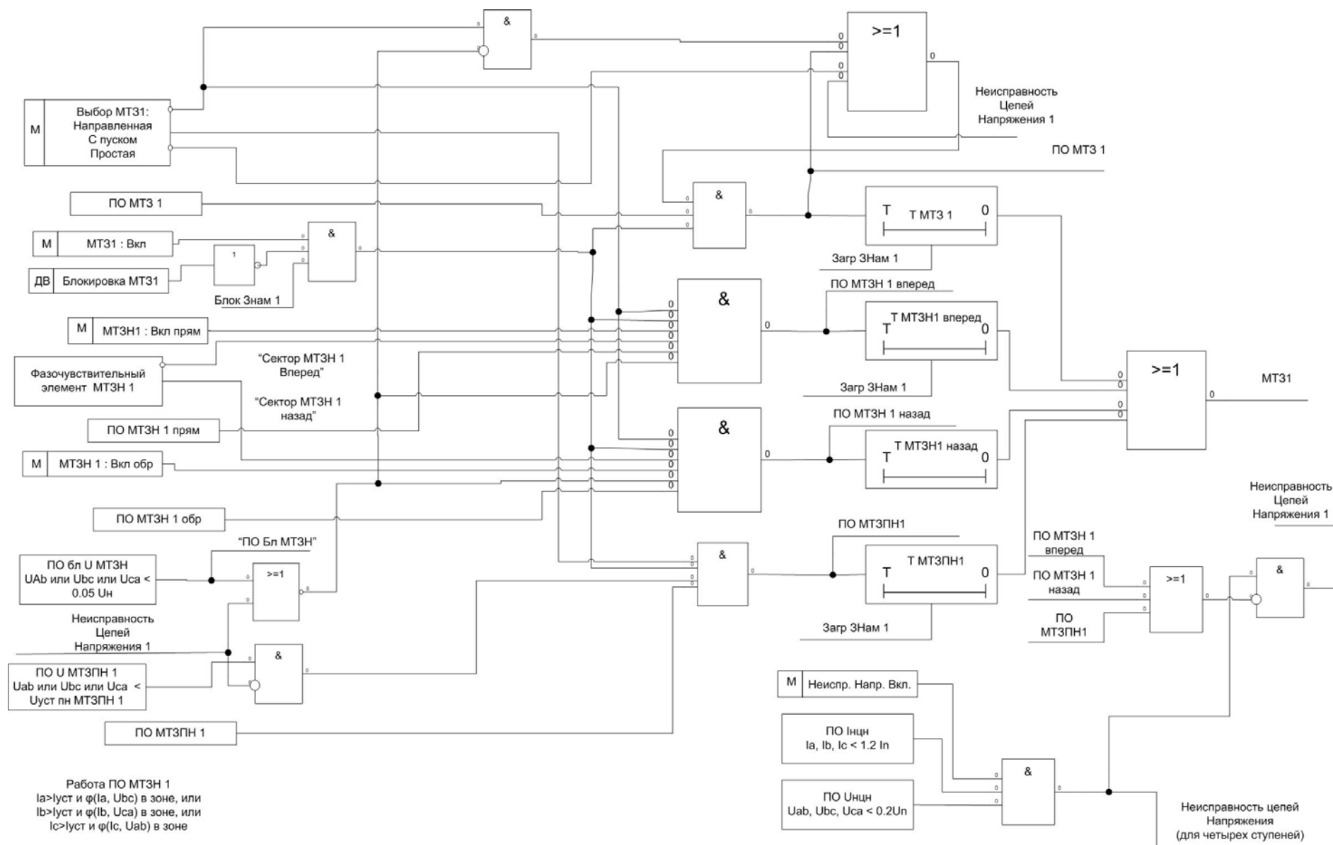
Рис. 1.7.2.2 Функциональная схема блока MT31
