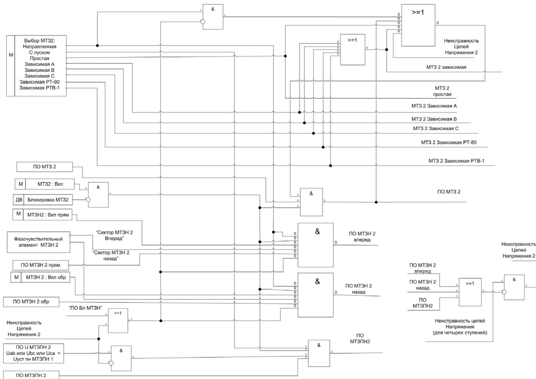
Рис. 1.7.2.3 Функциональная схема блока МТ32 (начало)
