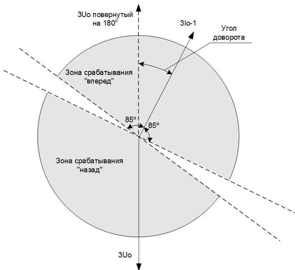
Рис. 1.7.15.1 Диаграмма направленности ТЗНП
