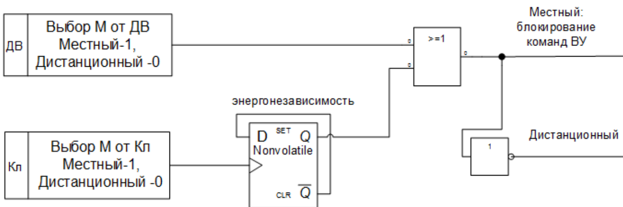
Рис.1.7.12 Функциональная схема блока местный/дистанционный режимы работы
