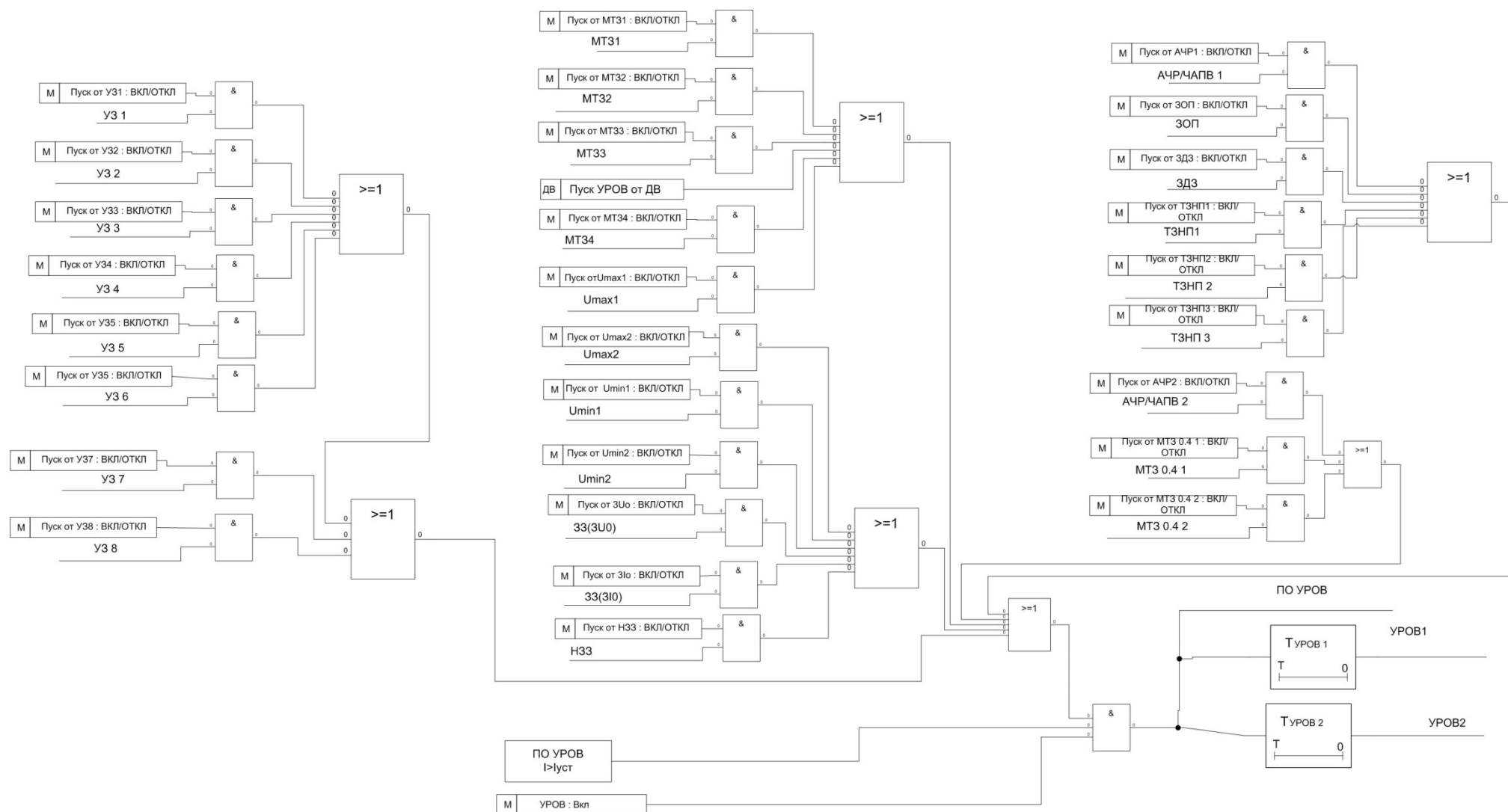
Рис. 1.7.9 Функциональная схема блока УРОВ
