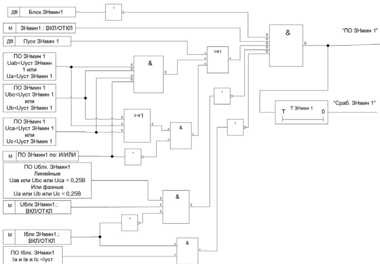
Рис.1.7.6 Функциональная схема блока ЗНмин1 (ЗНмин2 - идентично)
