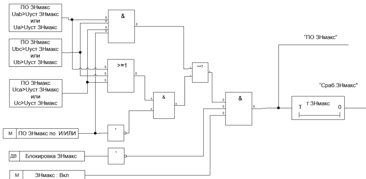
Рис.1.7.7 Функциональная схема блока ЗНмакс (алгоритмы работы первой и второй ступени идентичны)
