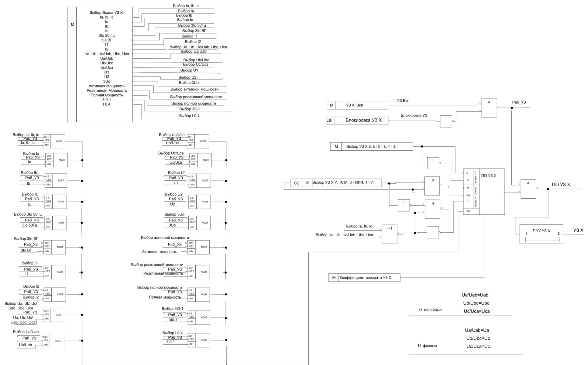
Рис. 1.7.25 Функциональная схема элемента универсальной защиты
