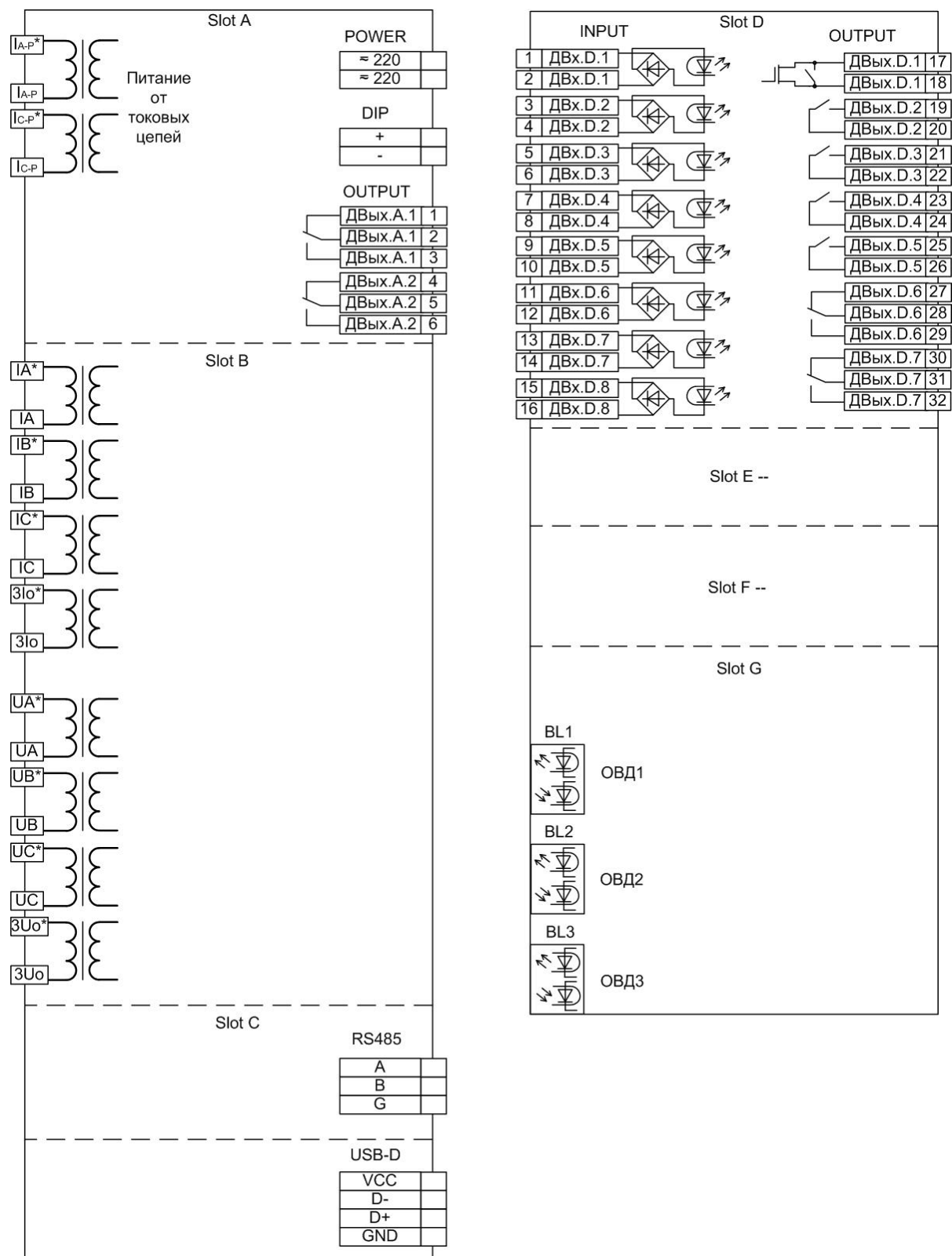
Рис. 2.1.2 Упрощенная схема подключения MZD-F (аппаратная конфигурация C)
