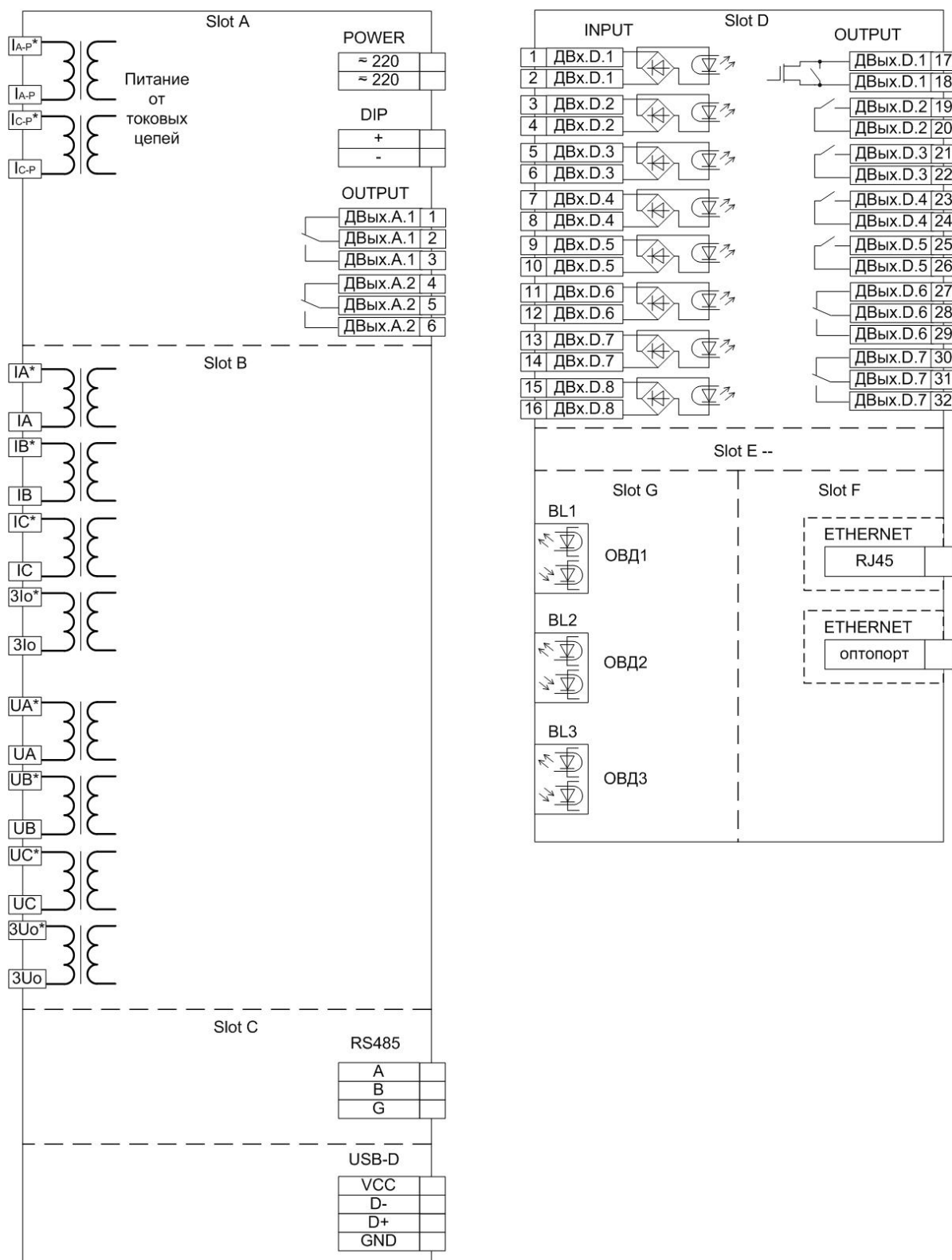
Рис. 2.1.3 Упрощенная схема подключения MZD-F (аппаратная конфигурация D)
