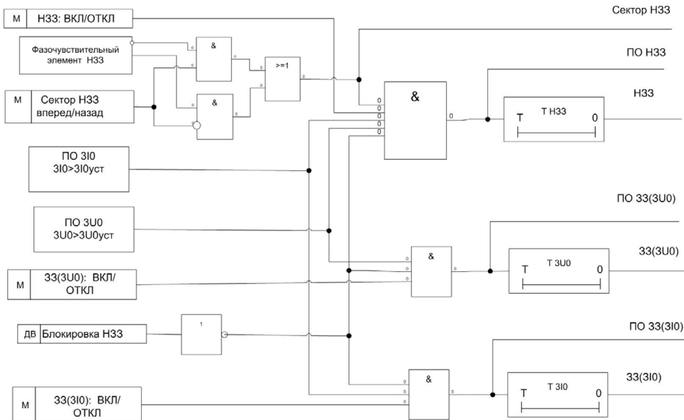
Рис. 1.7.3 Функциональная схема блоков защит от замыканий на землю по току, напряжению и направленной земляной защиты.
