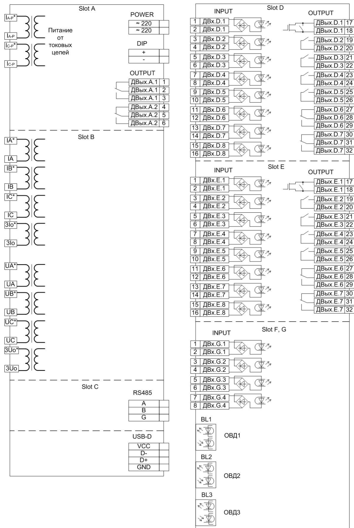
Рис. 2.1.6 Упрощенная схема подключения MZD-F (аппаратная конфигурация L)
