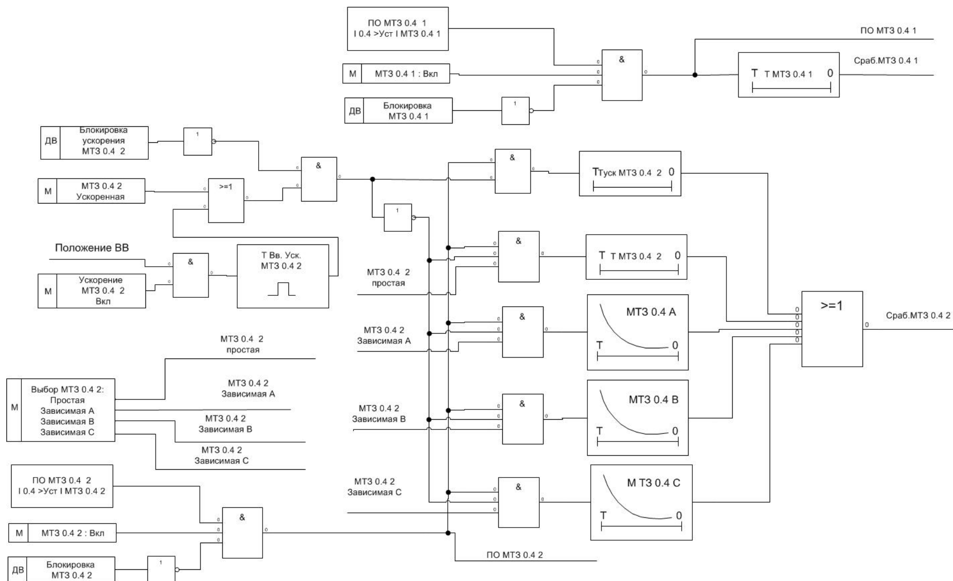
Рис. 1.7.16 Функциональная схема блока МТЗ 0.4
