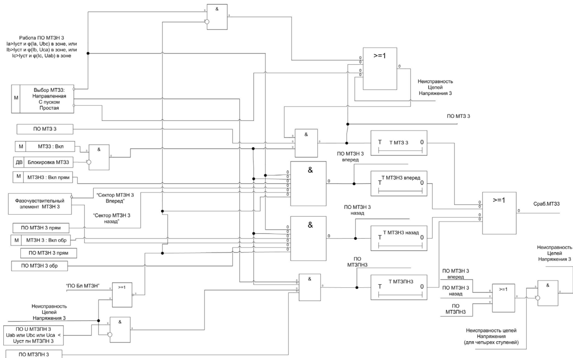
Рис. 1.7.2.5 Функциональная схема блока МТЗ3
